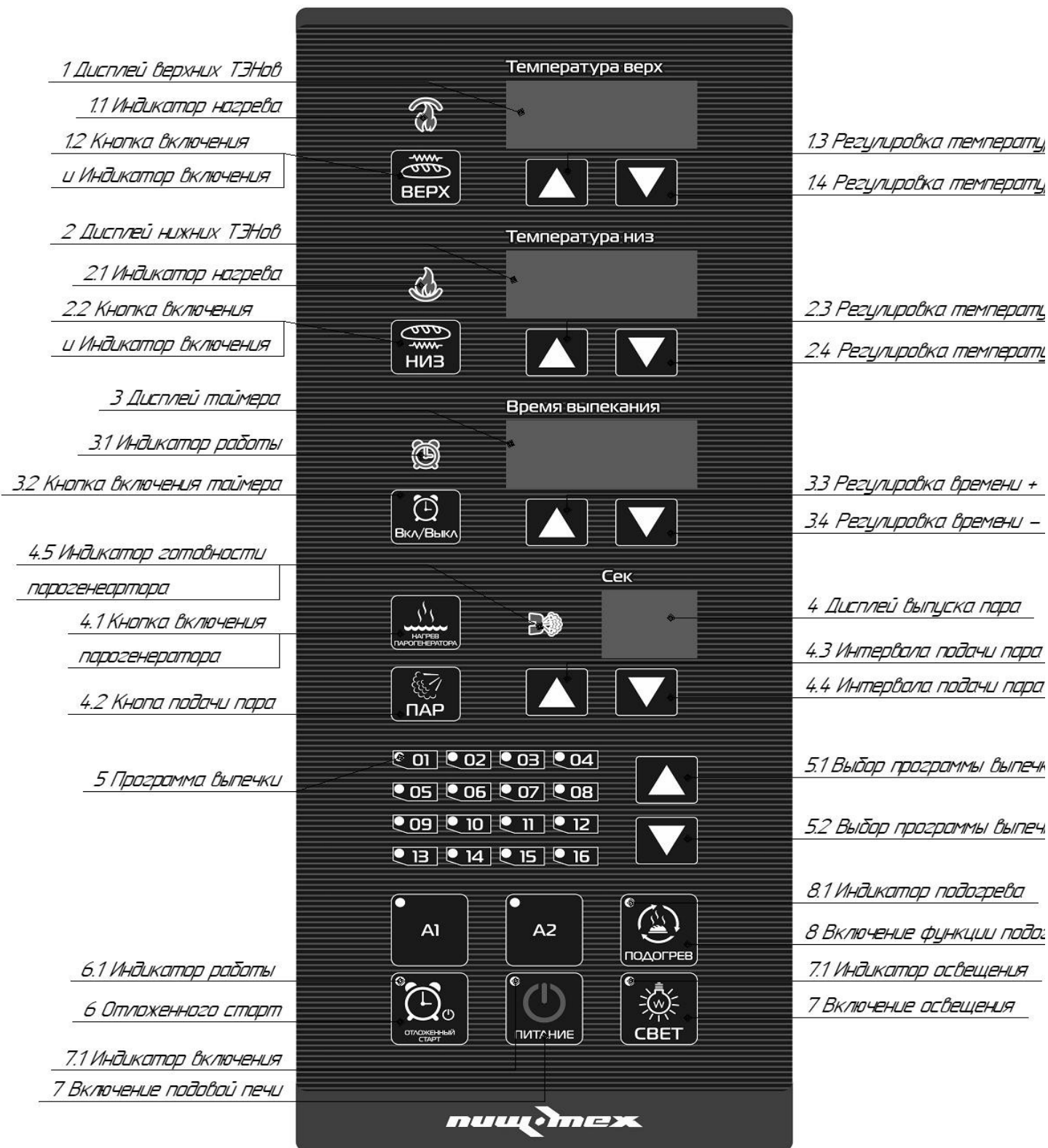
Рисунок 4 — Пульт ПОД-КП-Д
