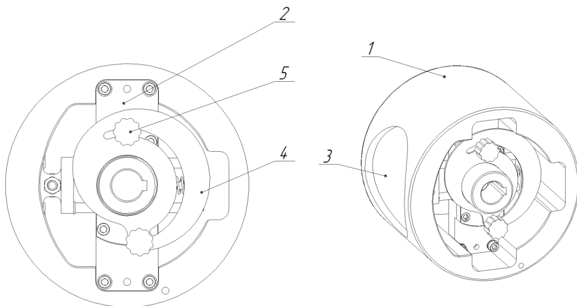
Рисунок 1. Устройство формующего барабана.
